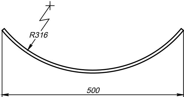
Поз.3 (Ложмент)
